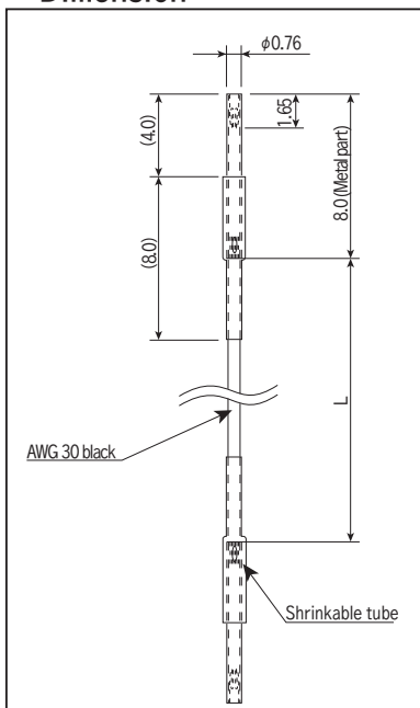
PRW-0.3-□
