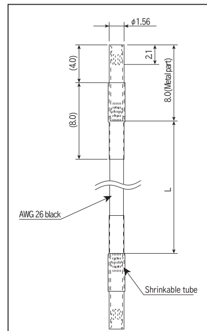
PRW-0.7-□
