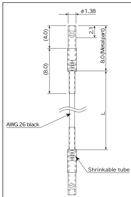
PRW-0.5-□
